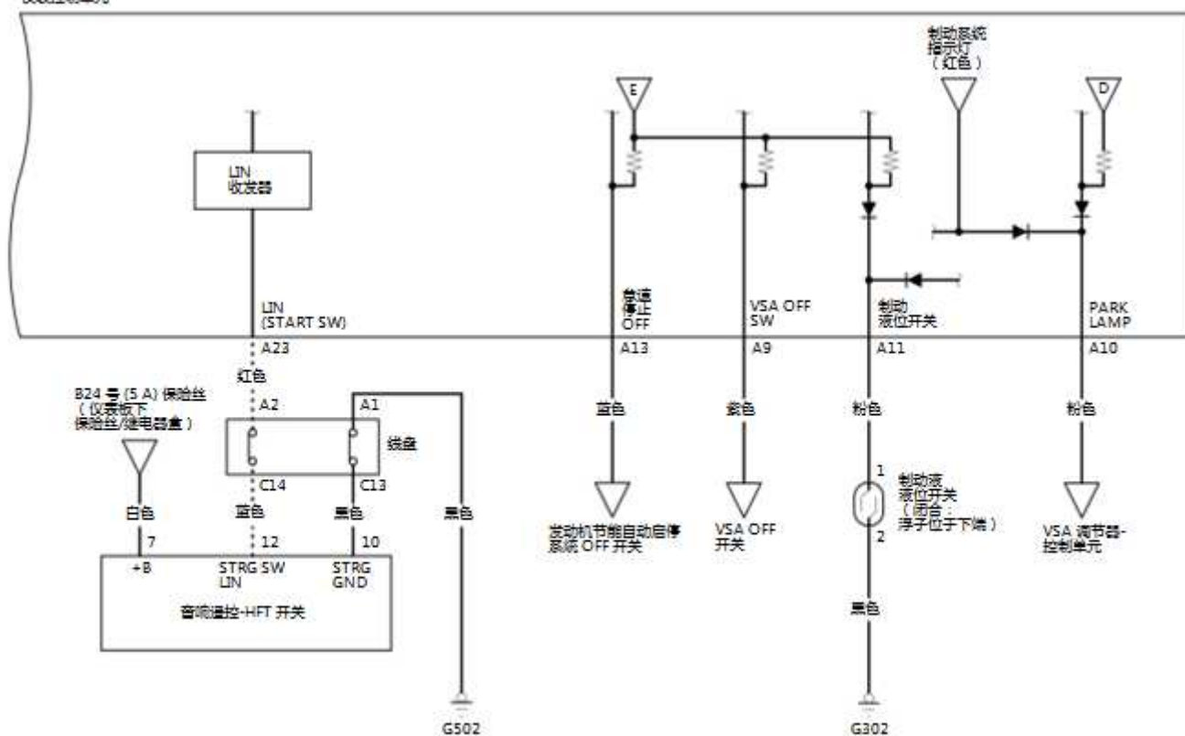
仪表控制单元
