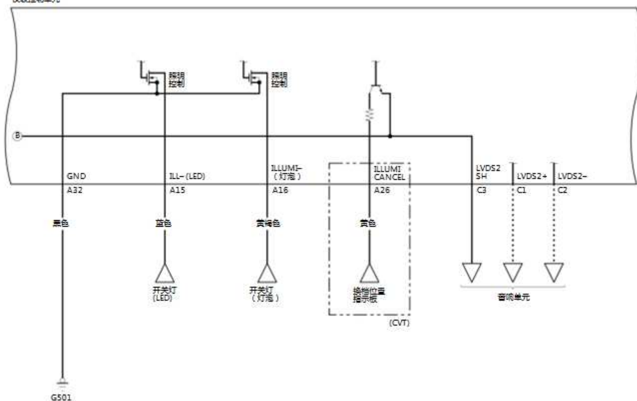
仪表控制单元
